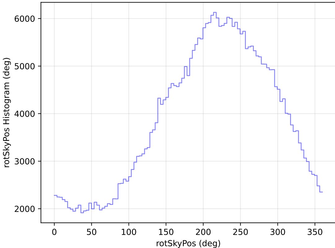
too_elab_r32_d2_ugrizy_v3.4_10yrs All sky y band: rotSkyPos Histogram
