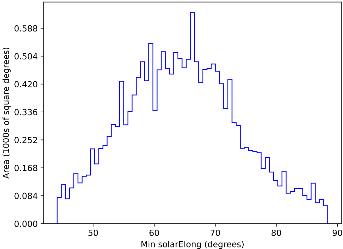
too_elab_r32_d2_ugrizy_v3.4_10yrs WFD y band: Min solarElong
