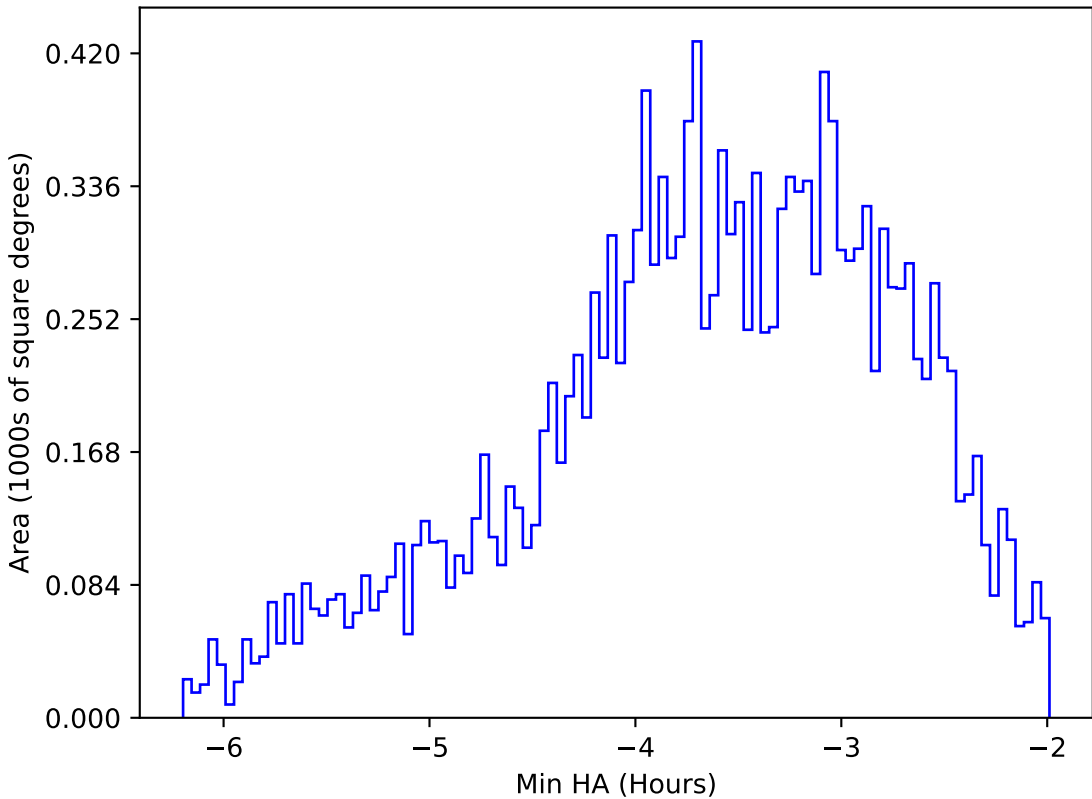
too_elab_r32_d2_ugrizy_v3.4_10yrs WFD y band: Min HA
