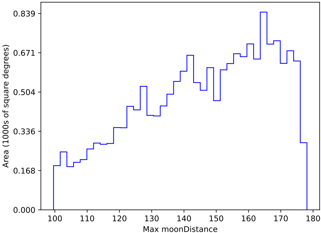
too_elab_r32_d2_ugrizy_v3.4_10yrs WFD y band: Max moonDistance
