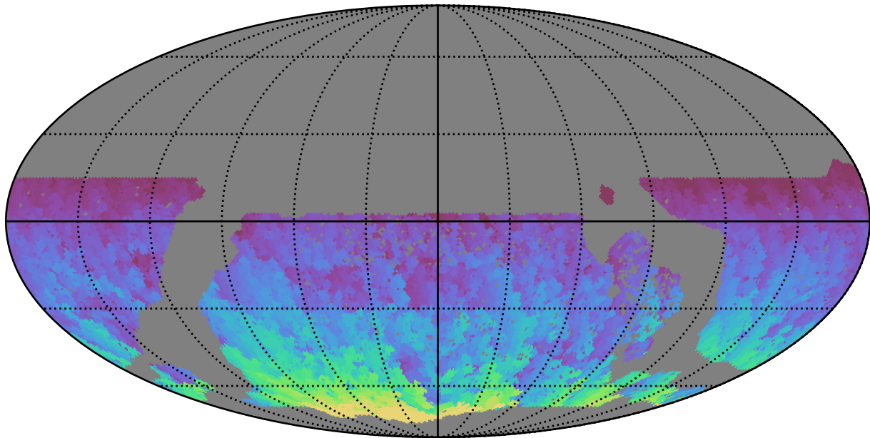
too_elab_r32_d2_ugrizy_v3.4_10yrs WFD y band: Max HA
