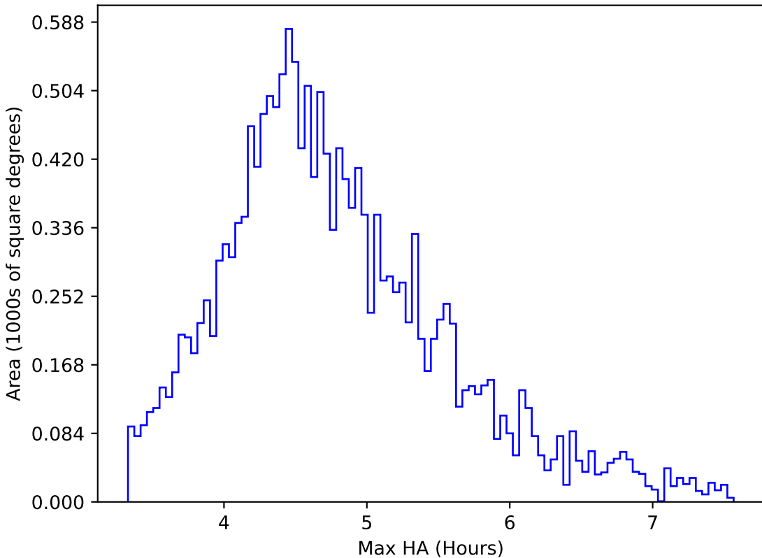
too_elab_r32_d2_ugrizy_v3.4_10yrs WFD y band: Max HA
