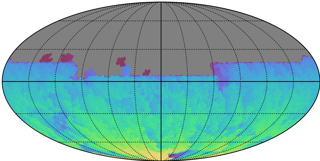
too_elab_r32_d2_ugrizy_v3.4_10yrs All sky y band: Max HA
