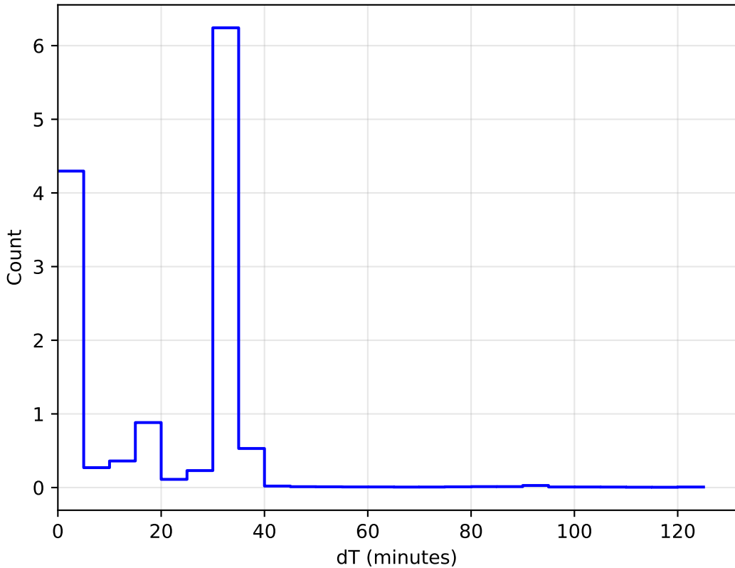
too_elab_r32_d2_ugrizy_v3.4_10yrs All sky: DeltaT Histogram 1e6
