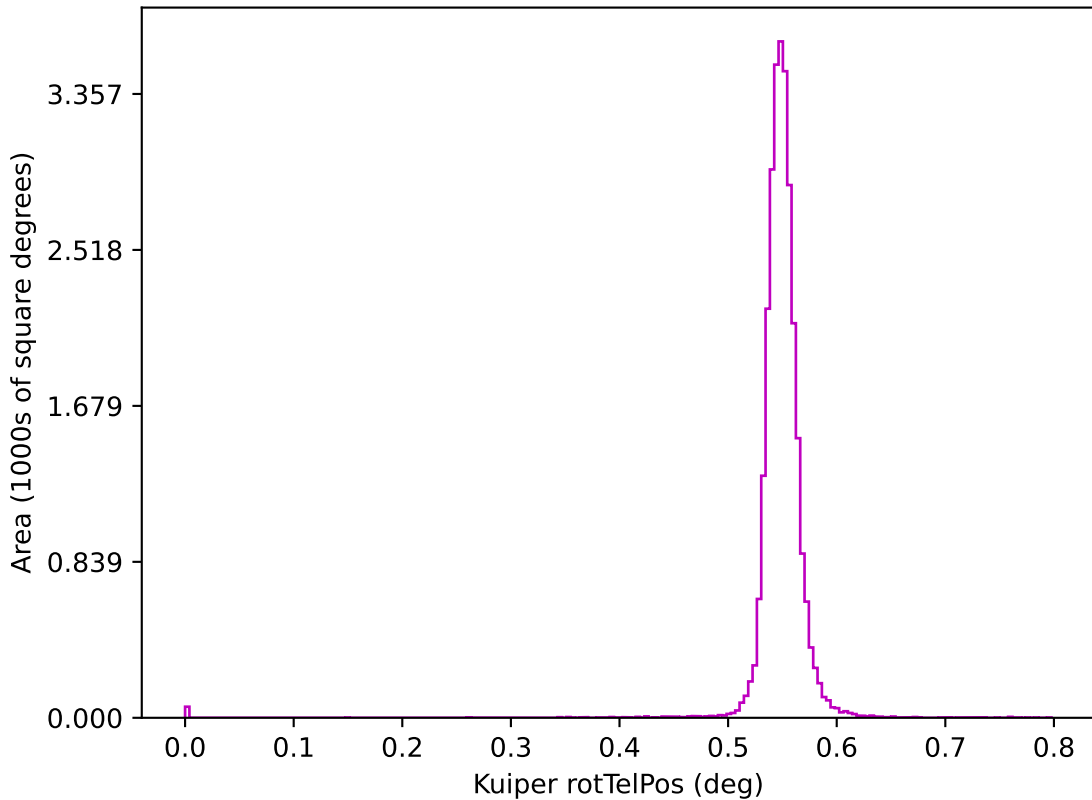
too_elab_r32_d2_gz_v3.4_10yrs z: Kuiper rotTelPos
