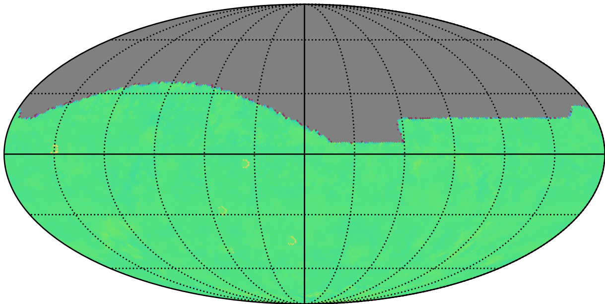
too_elab_r32_d2_gz_v3.4_10yrs i: Kuiper rotTelPos
