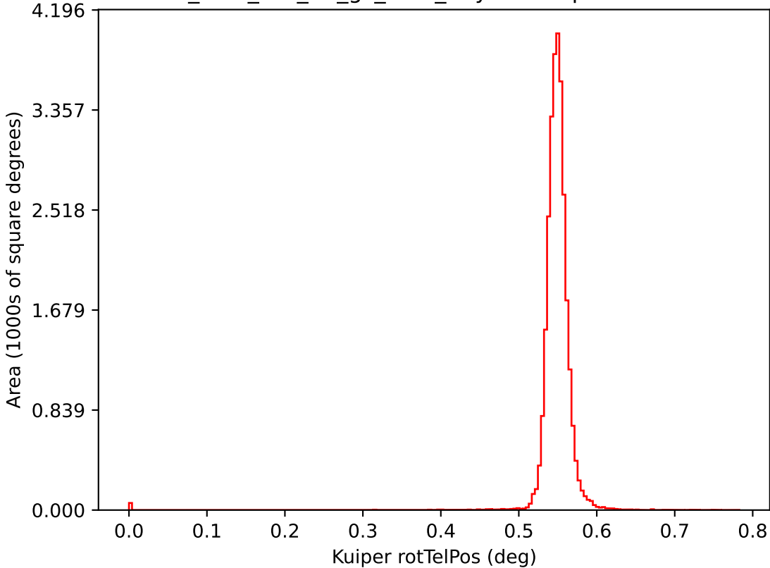
too_elab_r32_d2_gz_v3.4_10yrs i: Kuiper rotTelPos
