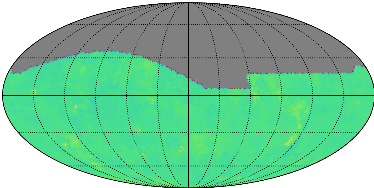
too_elab_r32_d2_gz_v3.4_10yrs g: Kuiper rotTelPos
