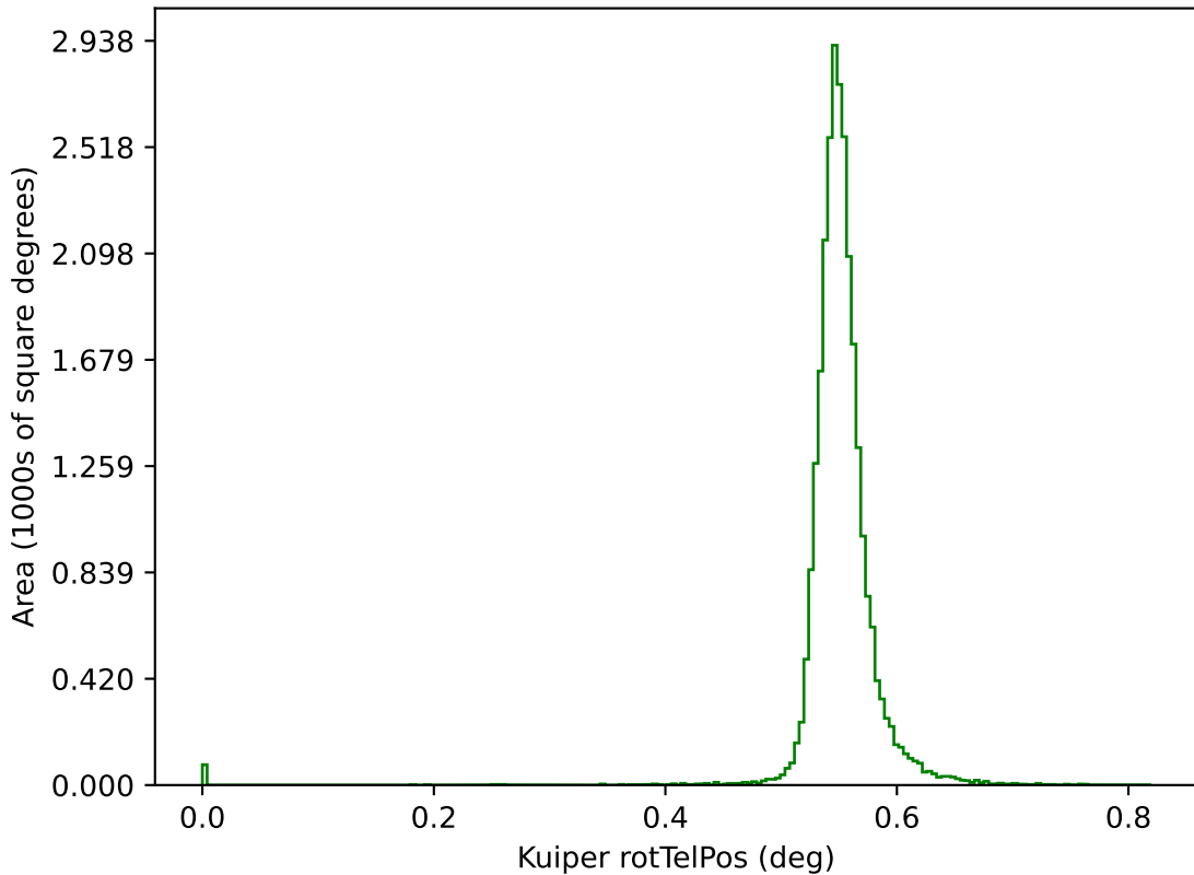
too_elab_r32_d2_gz_v3.4_10yrs g: Kuiper rotTelPos
