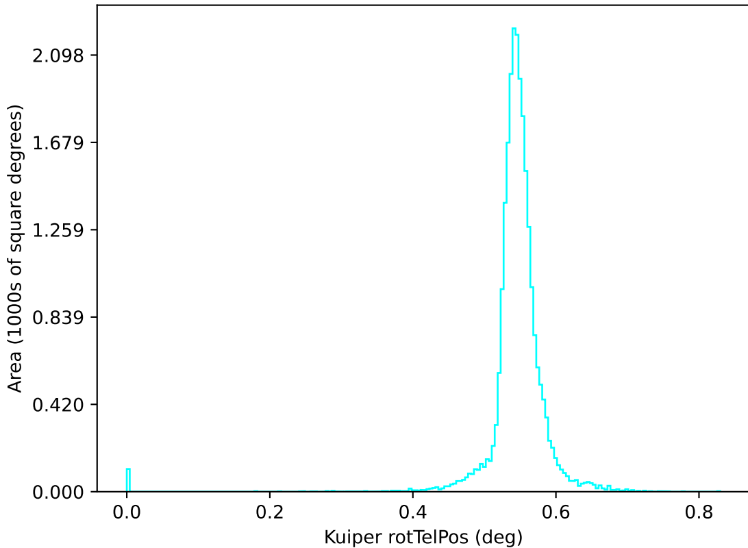
too_elab_r32_d2_griz_v3.4_10yrs u: Kuiper rotTelPos
