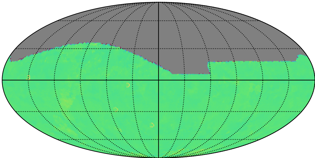
too_elab_r32_d2_griz_v3.4_10yrs i: Kuiper rotTelPos
