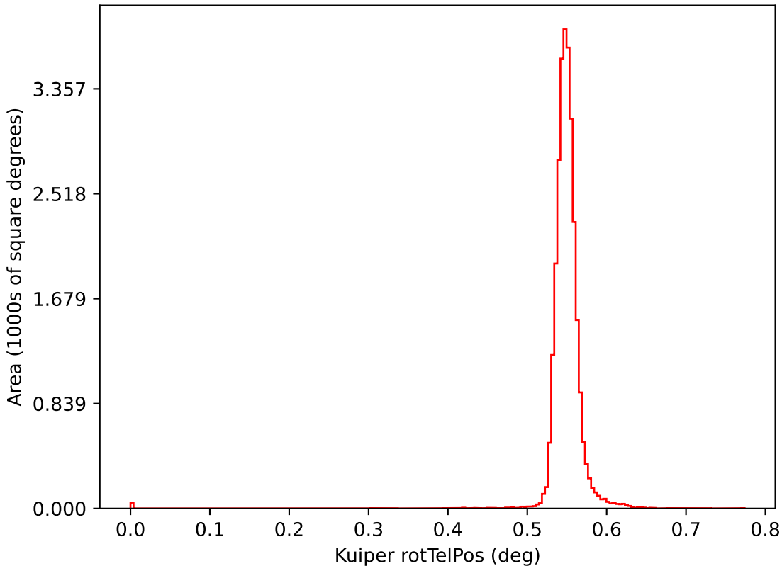
too_elab_r32_d2_griz_v3.4_10yrs i: Kuiper rotTelPos
