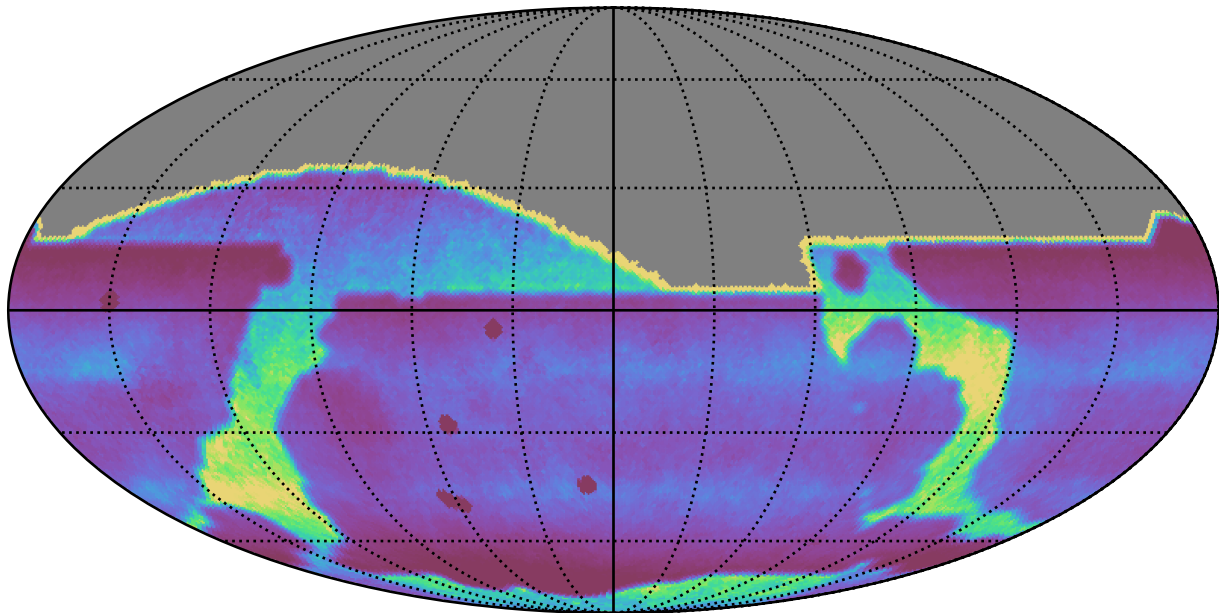
too_elab_r32_d2_griz_v3.4_10yrs : DCRprecision
