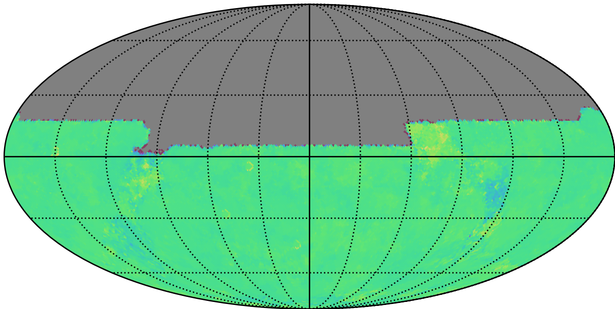
too_elab_r32_d2_giz_v3.4_10yrs u: Kuiper rotTelPos
