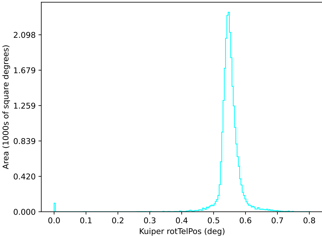
too_elab_r32_d2_giz_v3.4_10yrs u: Kuiper rotTelPos
