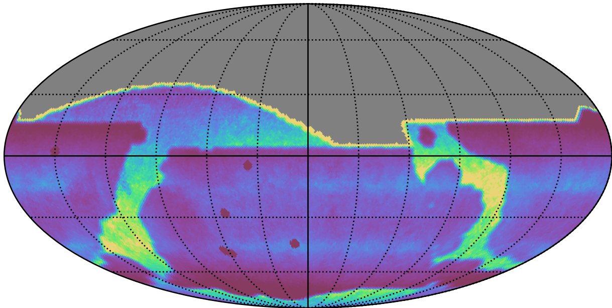
too_elab_r32_d2_giz_v3.4_10yrs : DCRprecision
