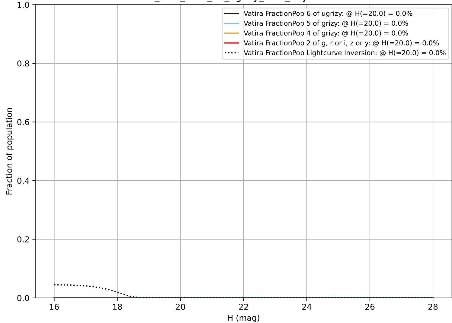
too_elab_r256_d3_ugrizy_v3.4_10yrs Vatira
