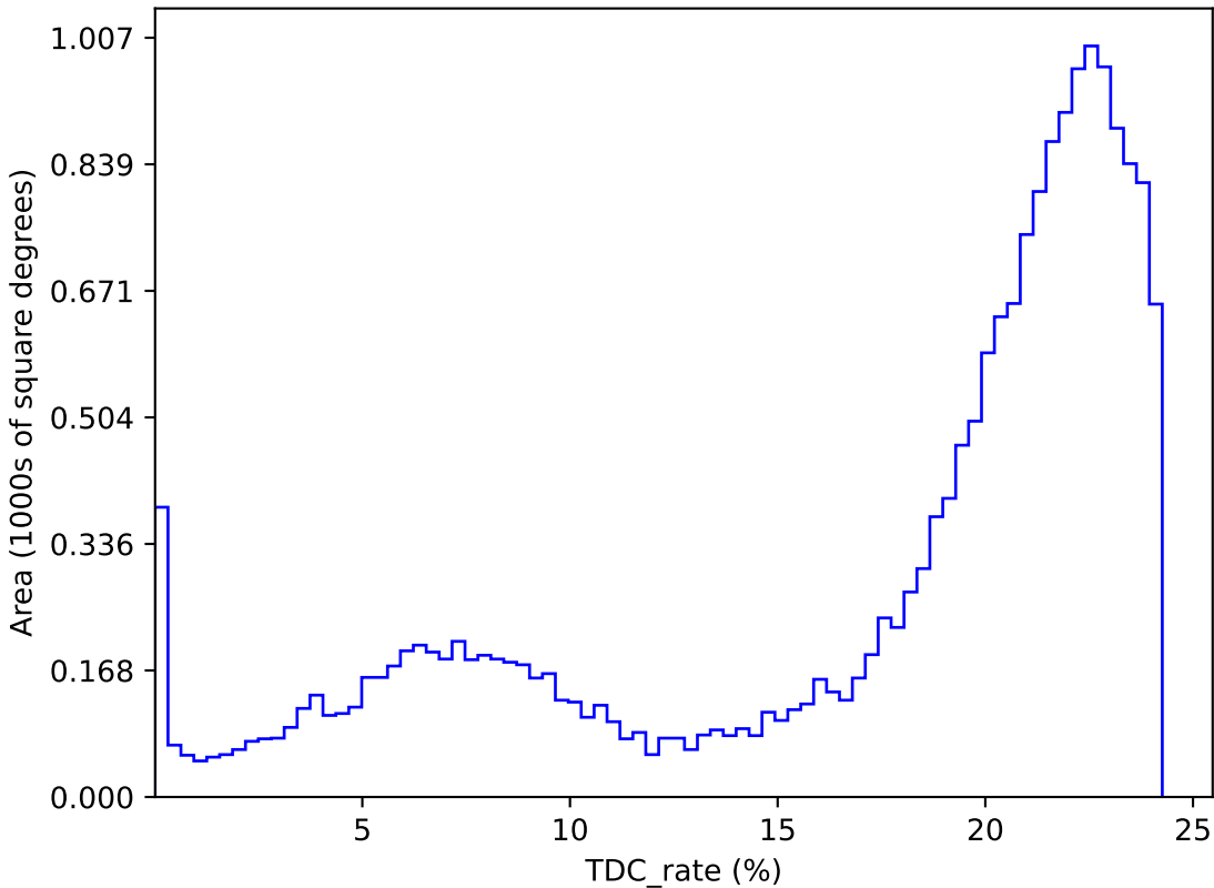
too_elab_r256_d3_ugrizy_v3.4_10yrs : TDC_rate
