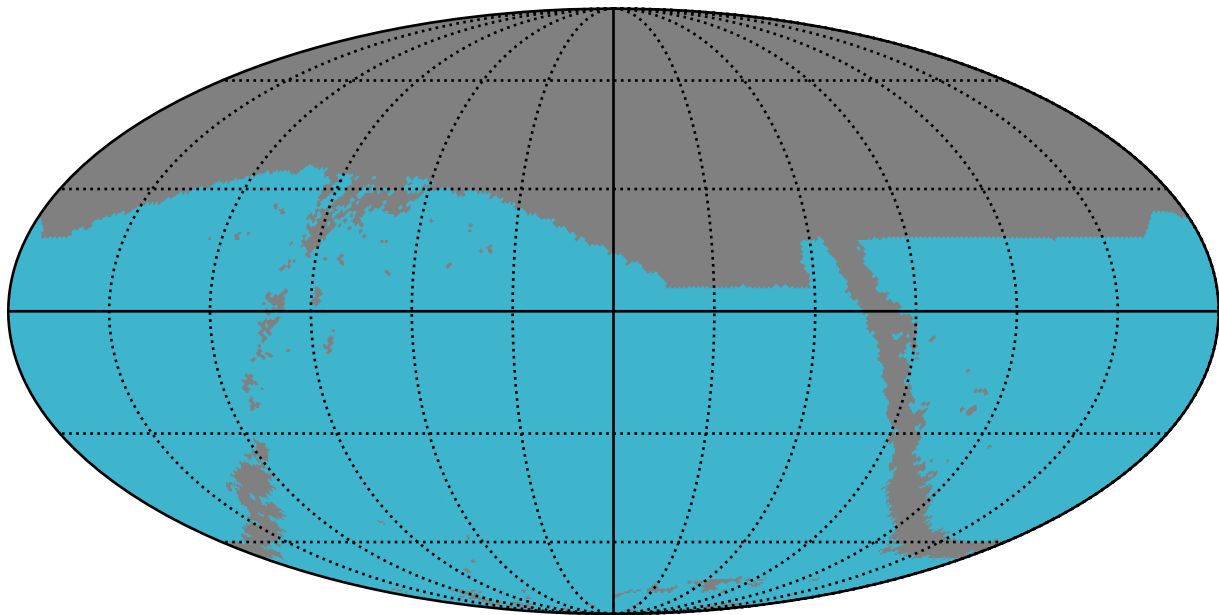
too_elab_r256_d3_ugrizy_v3.4_10yrs : SNSLMetric
