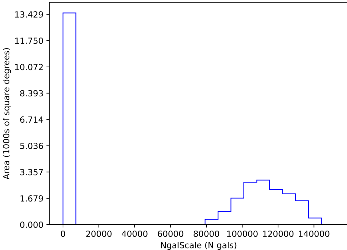
too_elab_r256_d3_ugrizy_v3.4_10yrs i: NgalScale
