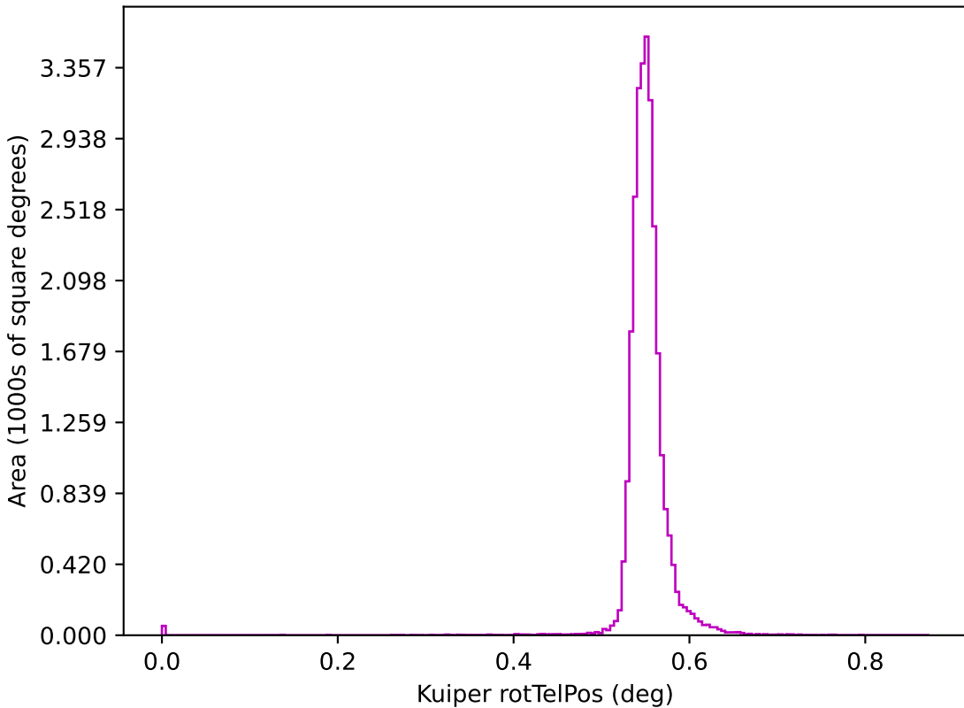
too_elab_r256_d3_ugrizy_v3.4_10yrs z: Kuiper rotTelPos
