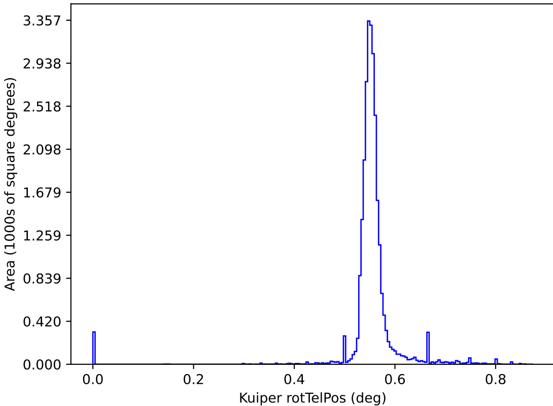
too_elab_r256_d3_ugrizy_v3.4_10yrs y: Kuiper rotTelPos
