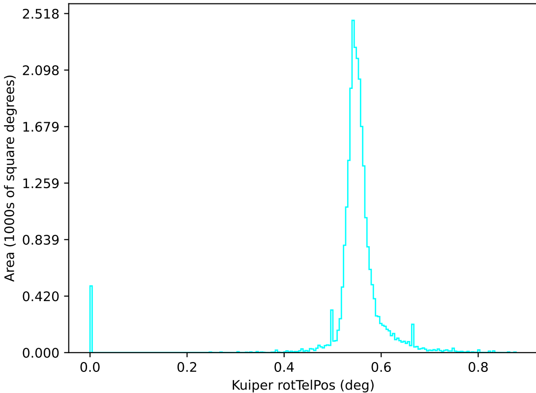
too_elab_r256_d3_ugrizy_v3.4_10yrs u: Kuiper rotTelPos
