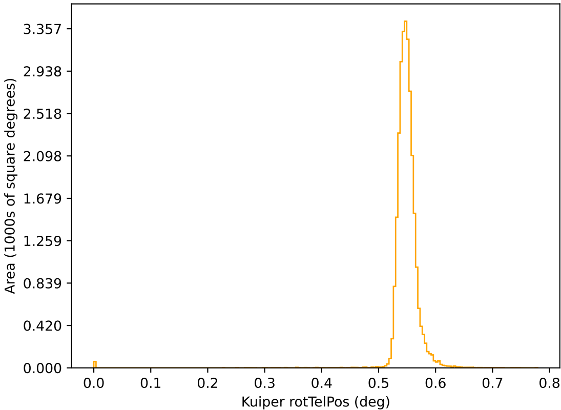
too_elab_r256_d3_ugrizy_v3.4_10yrs r: Kuiper rotTelPos
