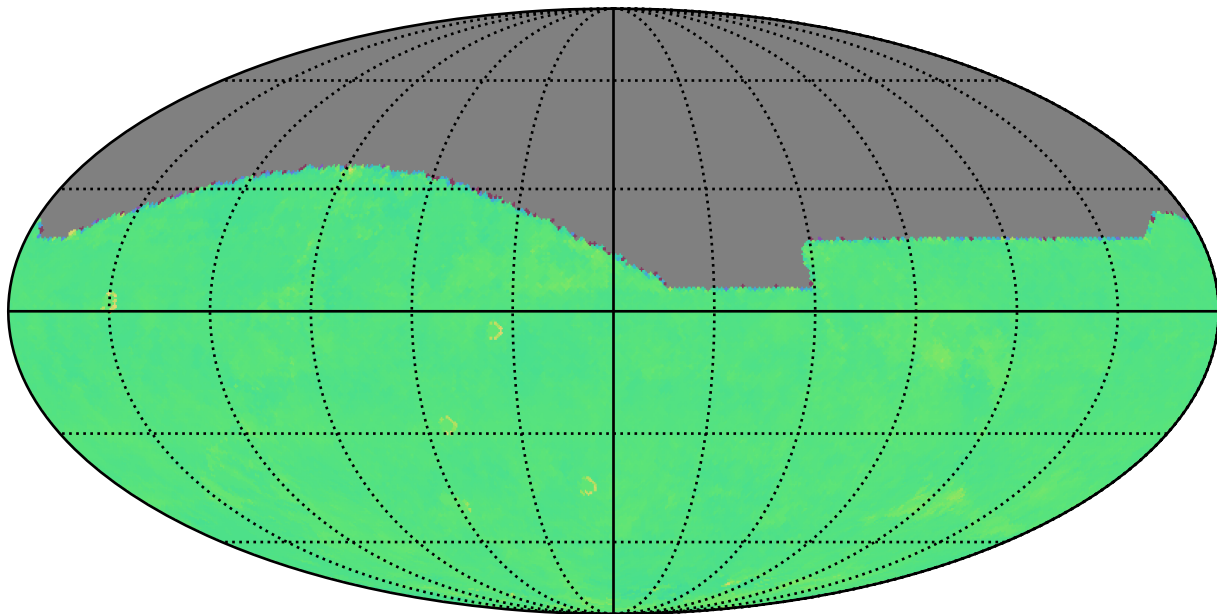
too_elab_r256_d3_ugrizy_v3.4_10yrs i: Kuiper rotTelPos
