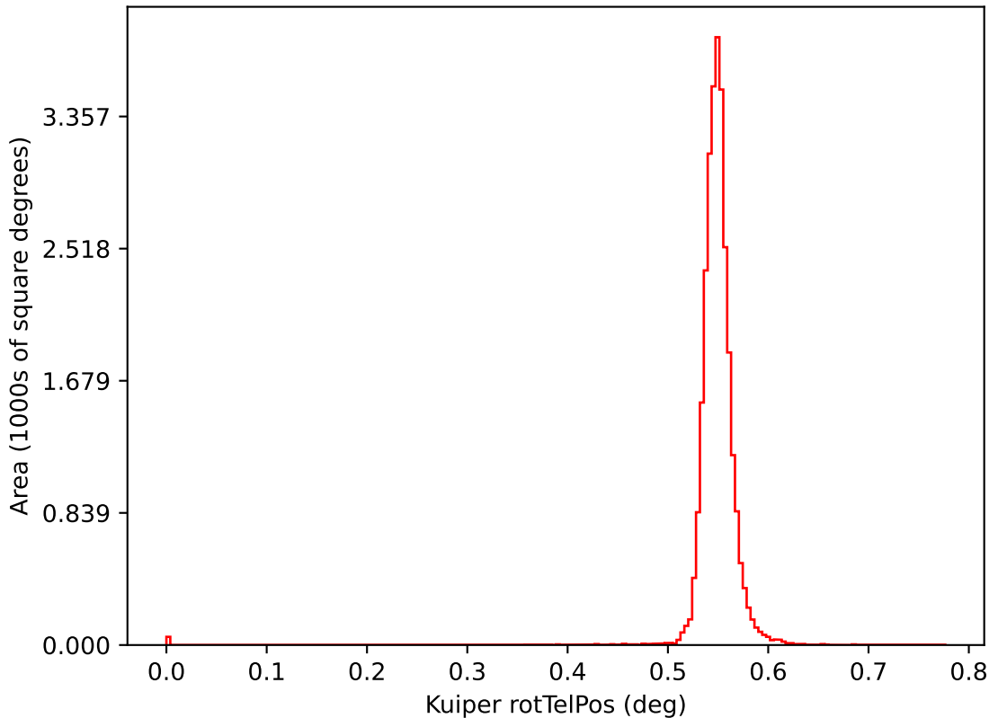
too_elab_r256_d3_ugrizy_v3.4_10yrs i: Kuiper rotTelPos
