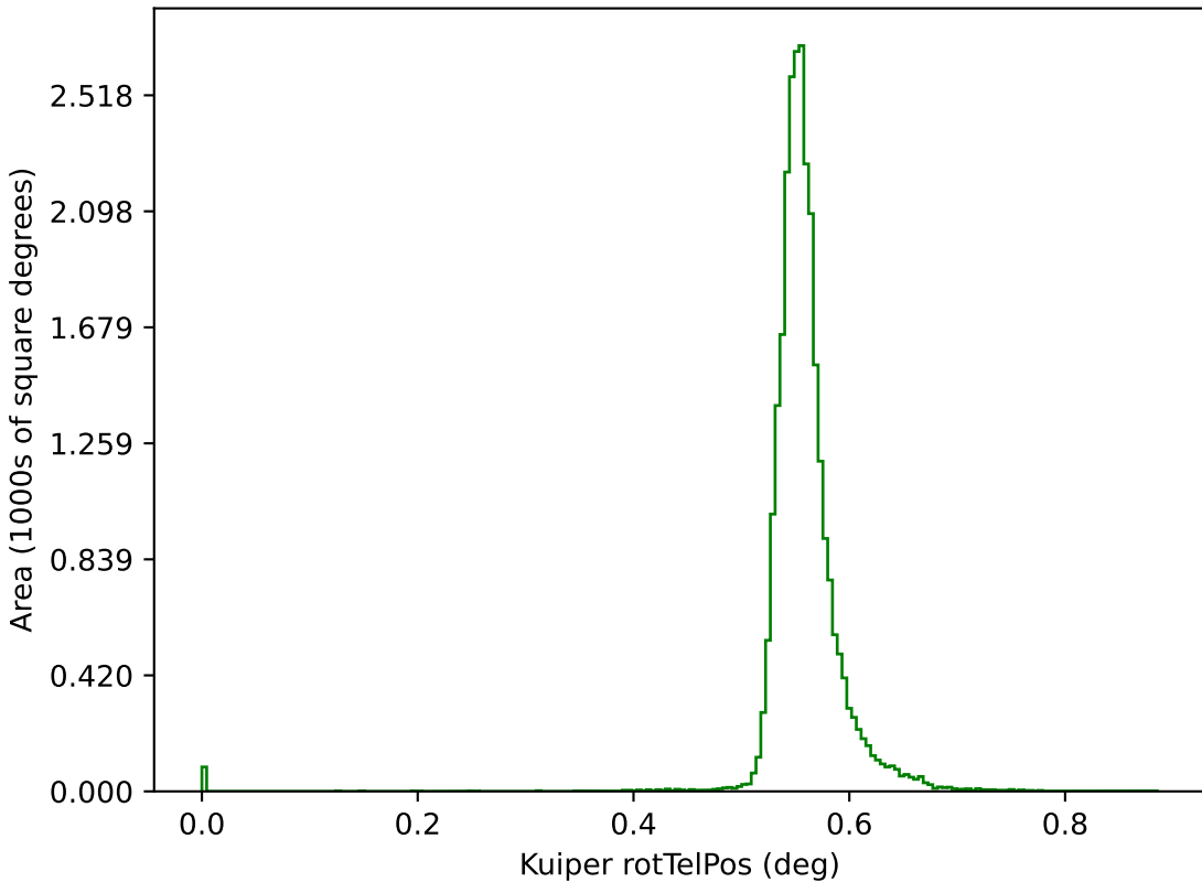
too_elab_r256_d3_ugrizy_v3.4_10yrs g: Kuiper rotTelPos
