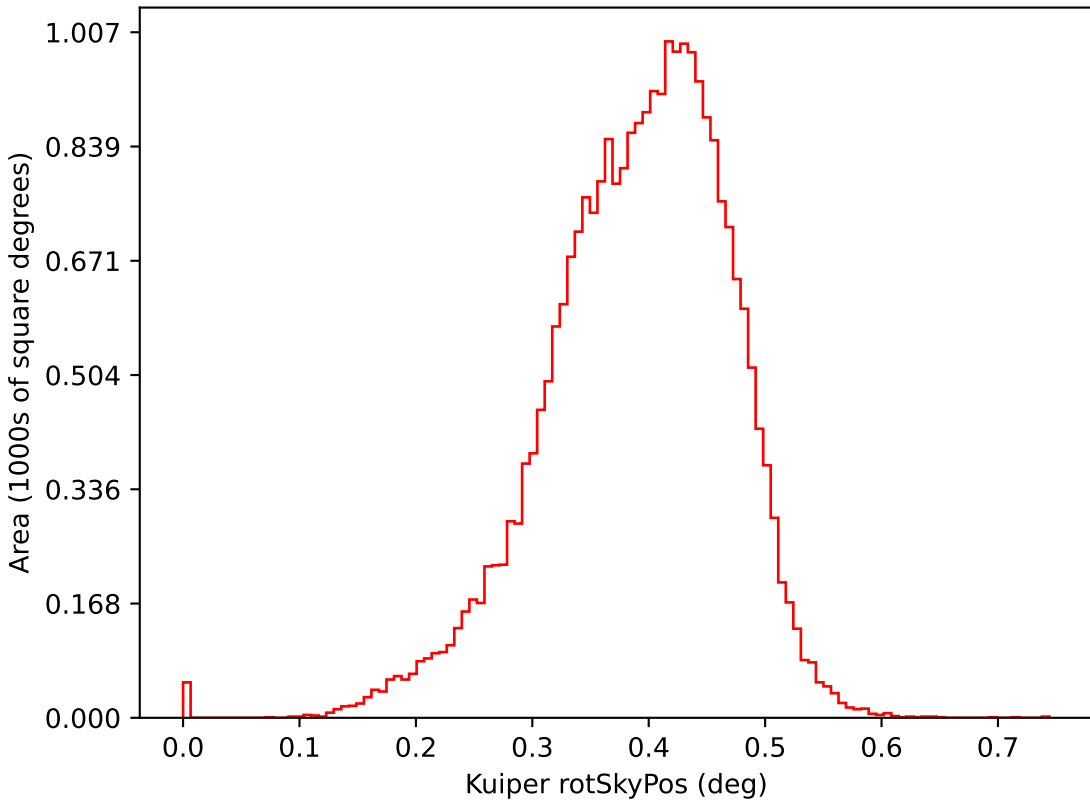
too_elab_r256_d3_ugrizy_v3.4_10yrs i: Kuiper rotSkyPos
