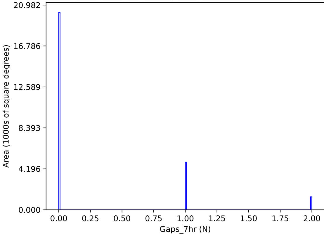
too_elab_r256_d3_ugrizy_v3.4_10yrs y band: Gaps_7hr
