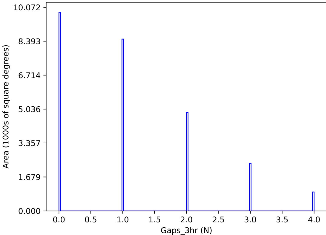
too_elab_r256_d3_ugrizy_v3.4_10yrs y band: Gaps_3hr
