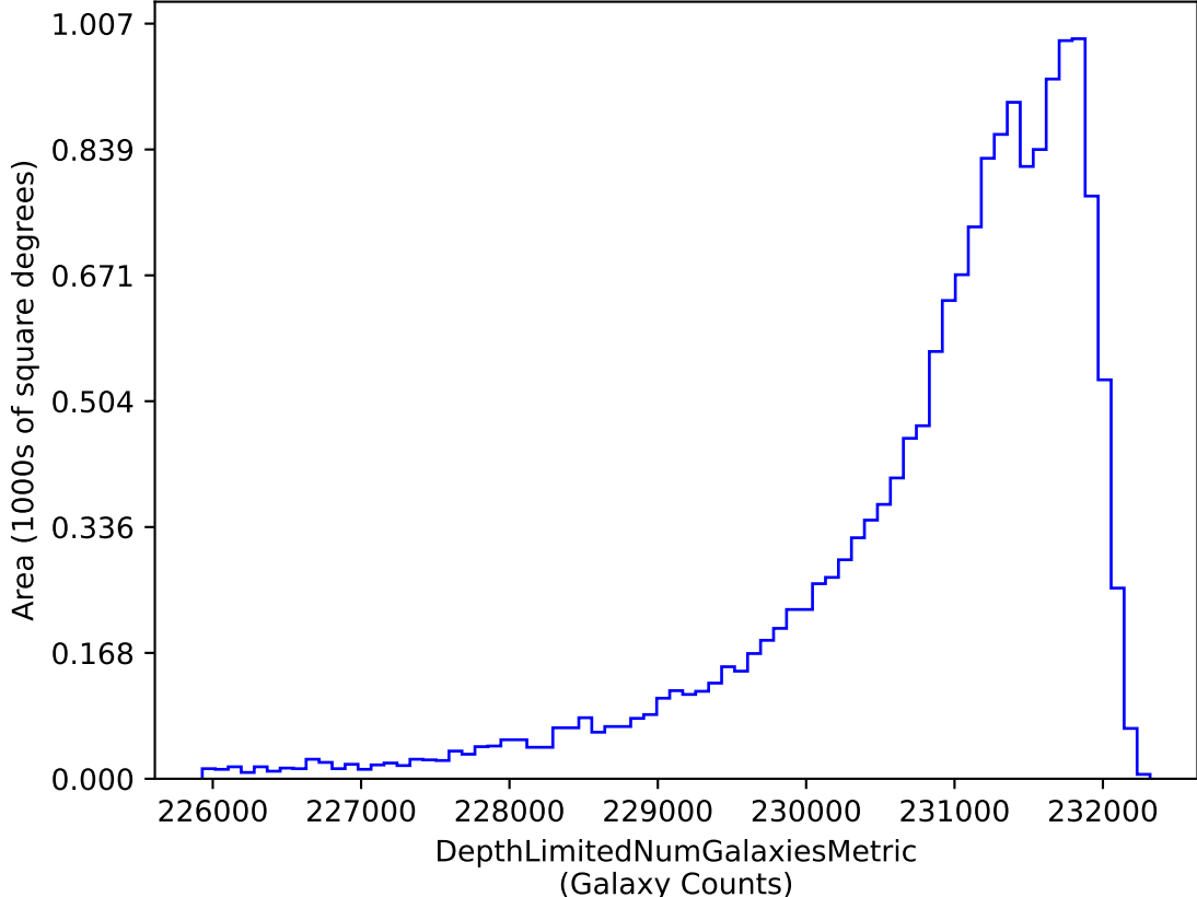
too_elab_r256_d3_ugrizy_v3.4_10yrs i band galaxies non-DD: DepthLimitedNumGalaxiesMetric
