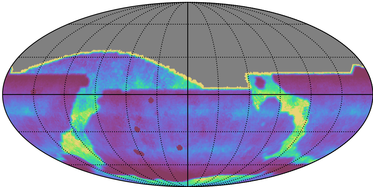
too_elab_r256_d3_ugrizy_v3.4_10yrs : DCRprecision
