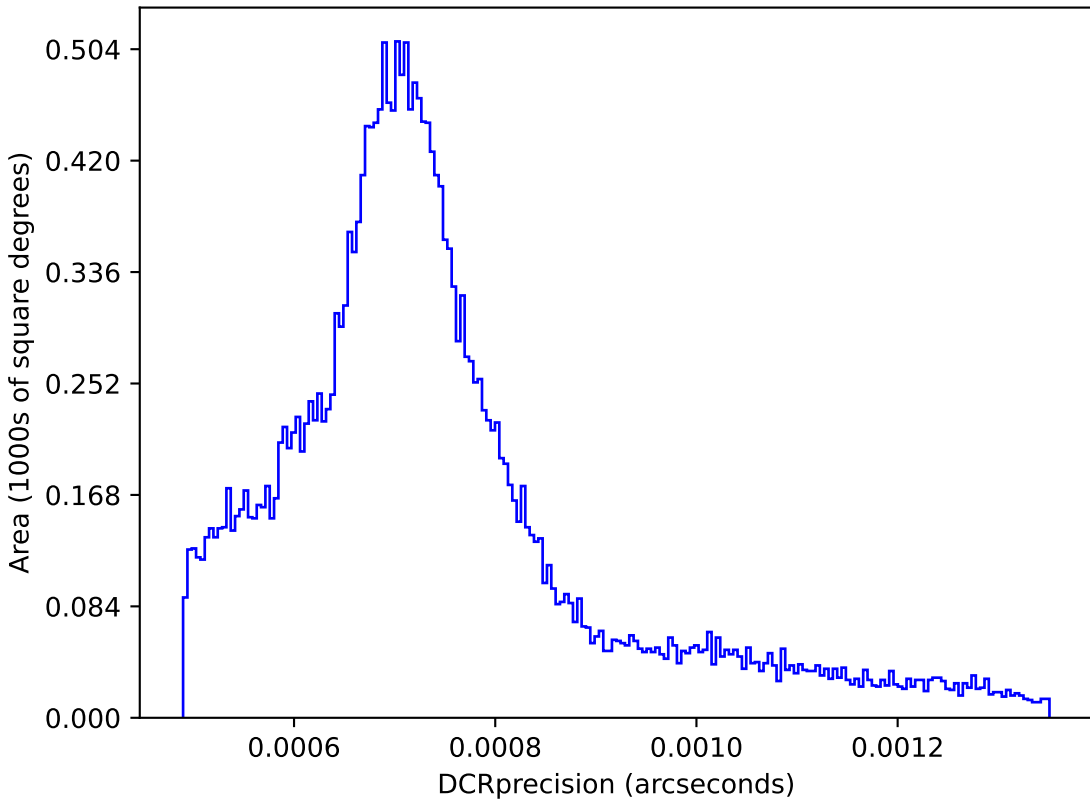
too_elab_r256_d3_ugrizy_v3.4_10yrs : DCRprecision
