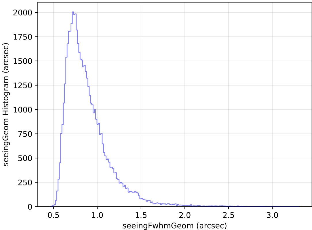
too_elab_r256_d3_ugrizy_v3.4_10yrs Yr 1 i band: seeingGeom Histogram
