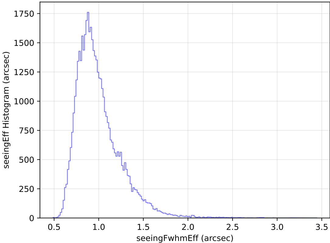
too_elab_r256_d3_ugrizy_v3.4_10yrs Yr 1 y band: seeingEff Histogram
