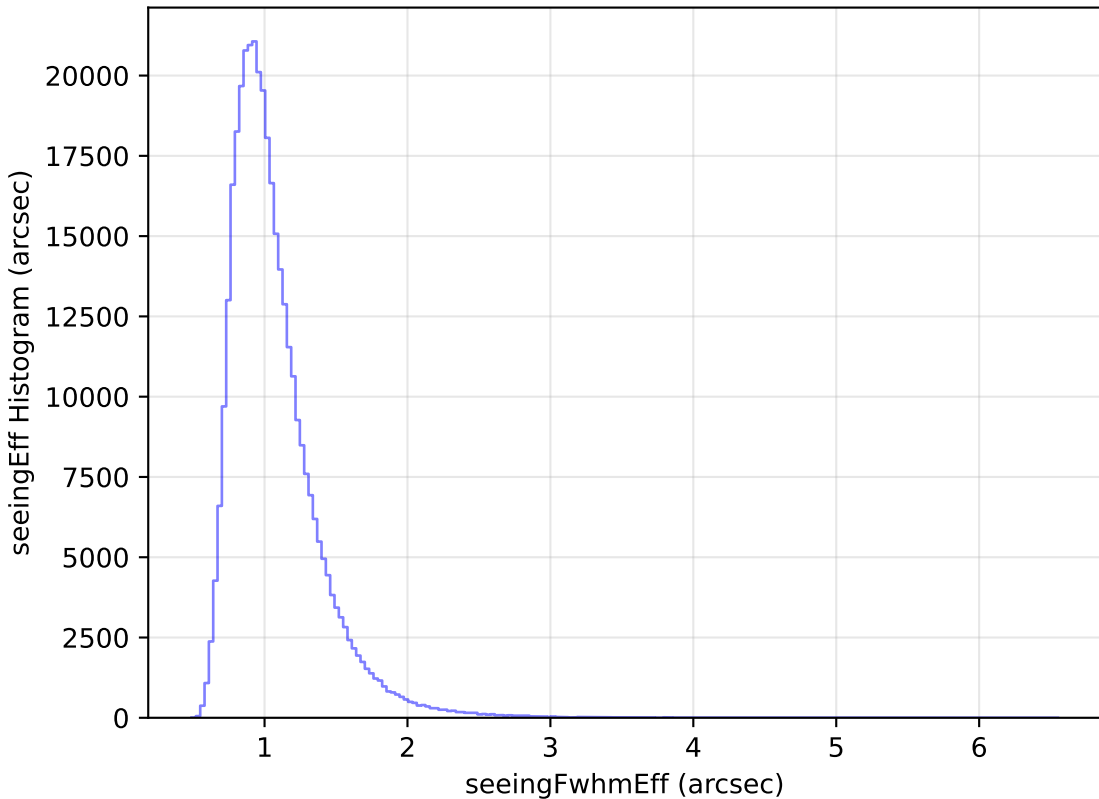
too_elab_r256_d3_ugrizy_v3.4_10yrs WFD y band: seeingEff Histogram
