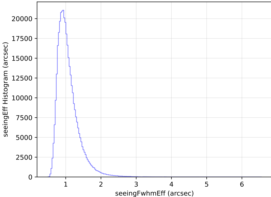
too_elab_r256_d3_ugrizy_v3.4_10yrs All sky y band: seeingEff Histogram
