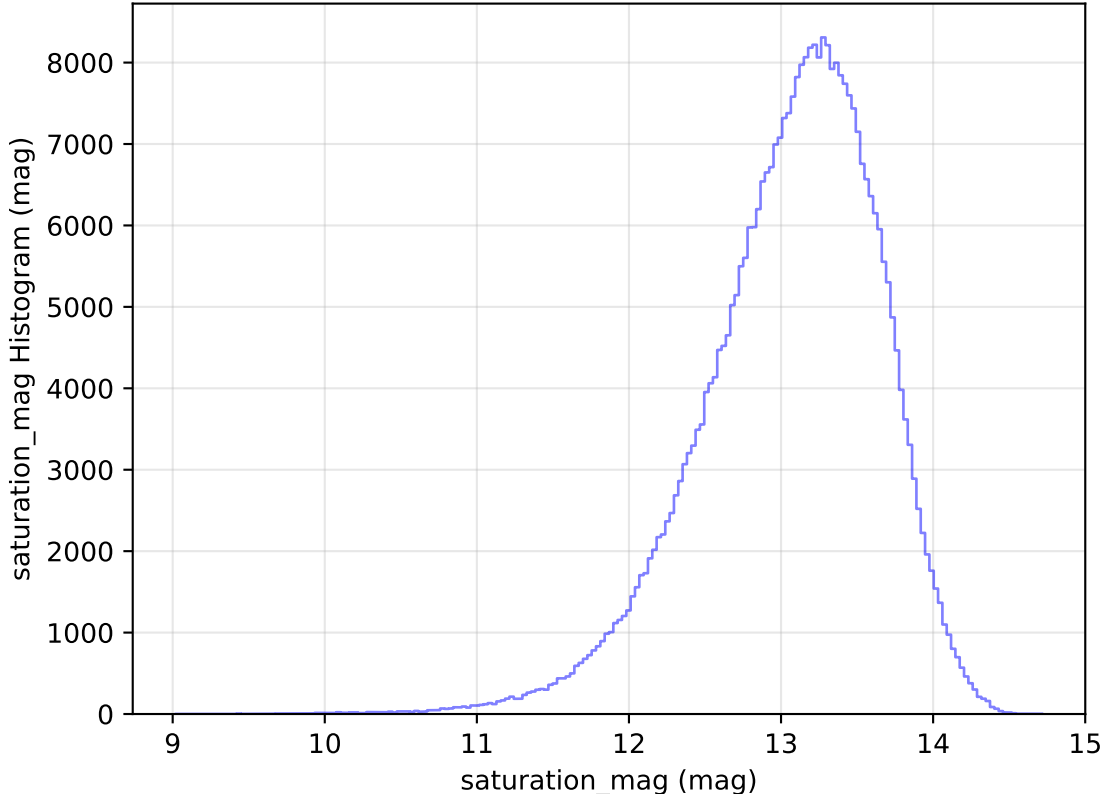
too_elab_r256_d3_ugrizy_v3.4_10yrs WFD y band: saturation_mag Histogram
