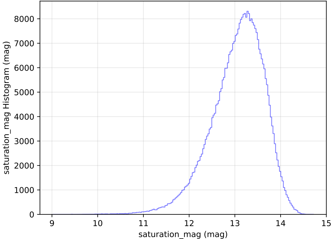
too_elab_r256_d3_ugrizy_v3.4_10yrs All sky y band: saturation_mag Histogram
