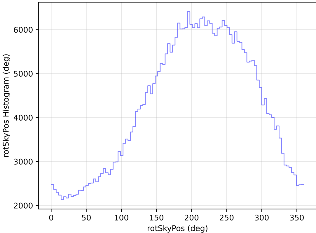
too_elab_r256_d3_ugrizy_v3.4_10yrs WFD z band: rotSkyPos Histogram
