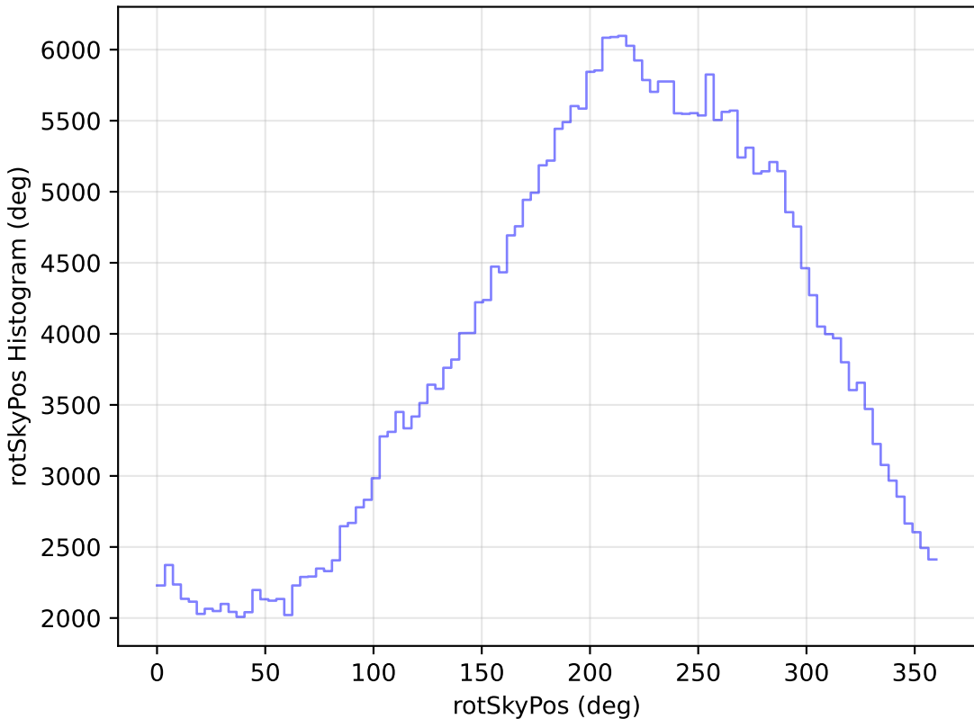
too_elab_r256_d3_ugrizy_v3.4_10yrs WFD y band: rotSkyPos Histogram
