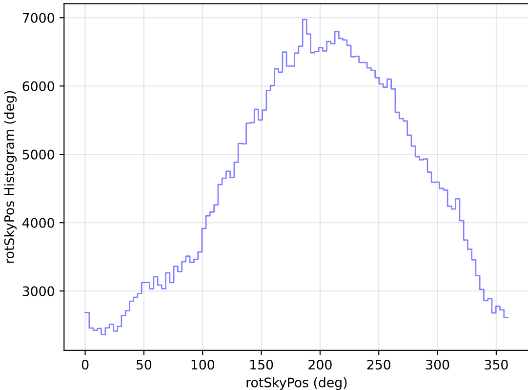
too_elab_r256_d3_ugrizy_v3.4_10yrs WFD r band: rotSkyPos Histogram
