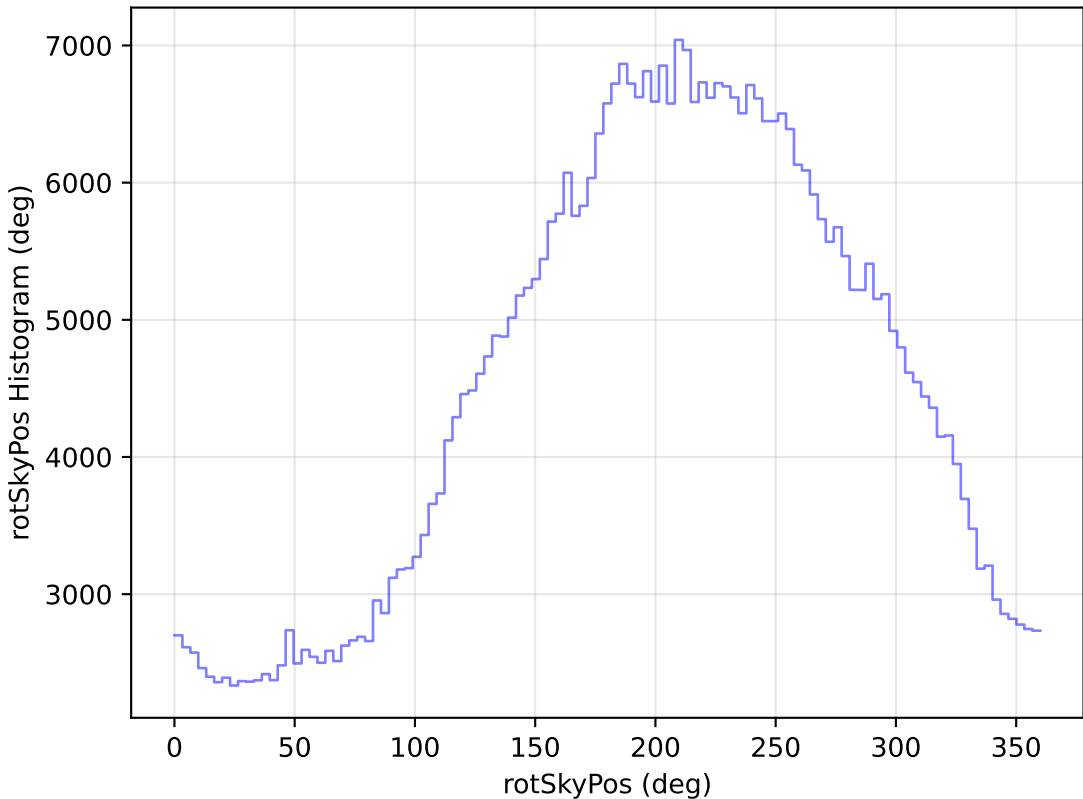
too_elab_r256_d3_ugrizy_v3.4_10yrs WFD i band: rotSkyPos Histogram
