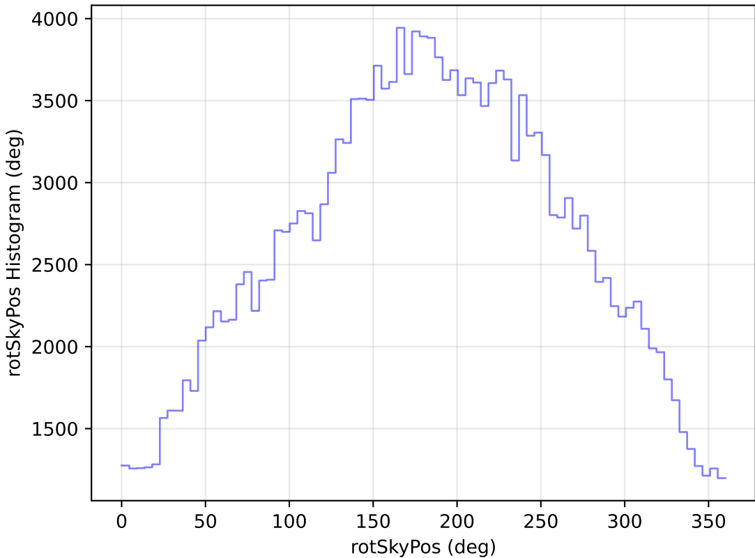
too_elab_r256_d3_ugrizy_v3.4_10yrs WFD g band: rotSkyPos Histogram
