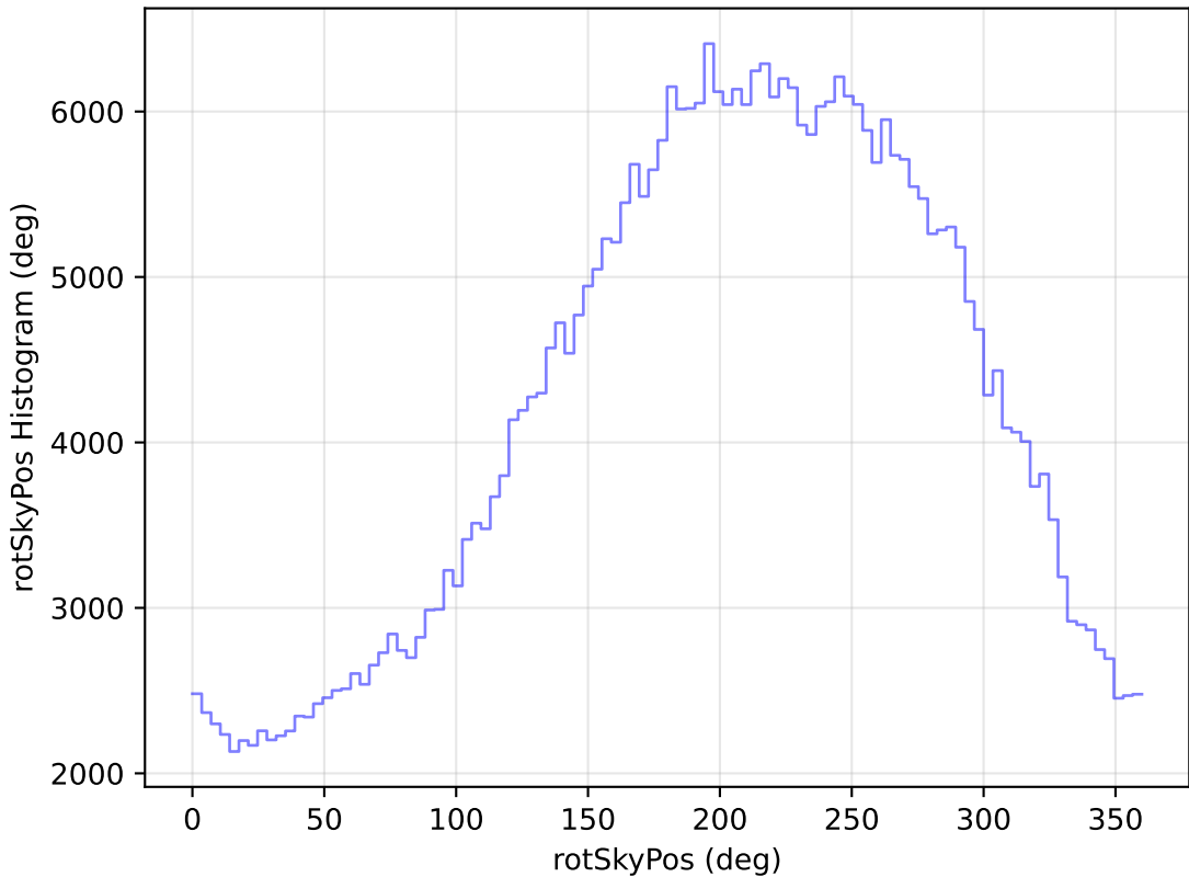
too_elab_r256_d3_ugrizy_v3.4_10yrs All sky z band: rotSkyPos Histogram
