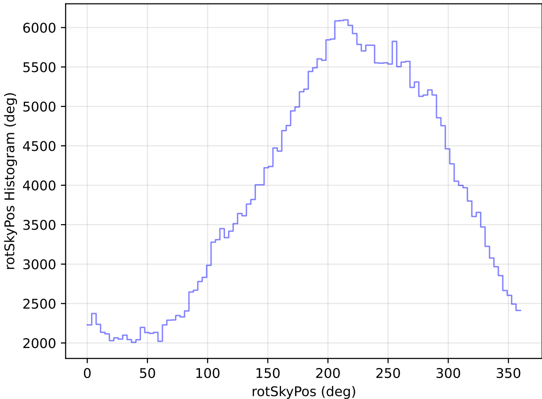
too_elab_r256_d3_ugrizy_v3.4_10yrs All sky y band: rotSkyPos Histogram
